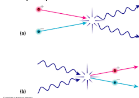
Figura 38: Ilustração da produção de pares e aniquilação.
