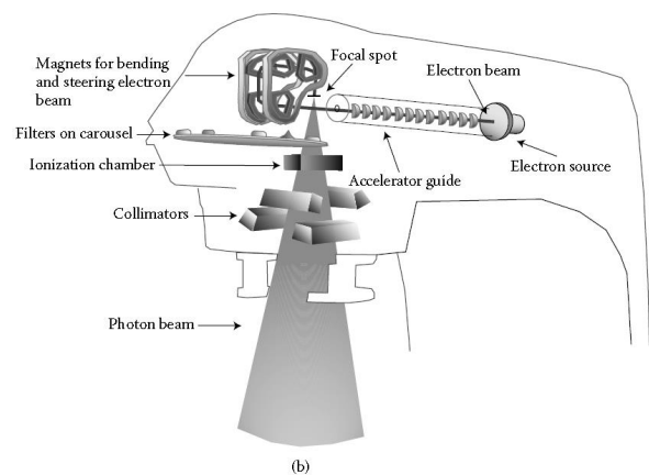
Figura 16: Fotografia do acelerador linear e composições internas do acelerador.
