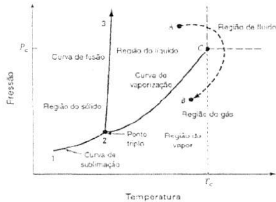
Figura 1 – Diagrama de fase de um fluido como a água.
