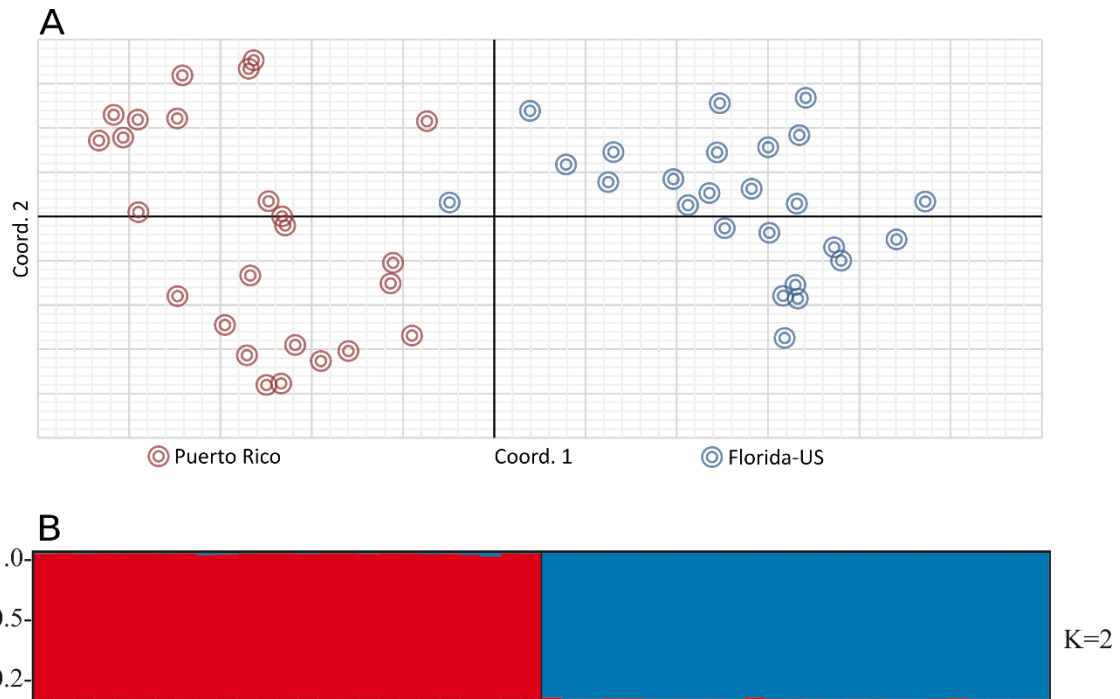
FIGURA 1. (A) Scatter-plot análise de coordenadas principais (PCoA) usando locos microssatélites C. guanhumii (B) Estrutura genética de populações de Cardisoma guanhumii baseada na análise Bayesiana do software Structure (K=2). Os indivíduos são representados em cada linha vertical
