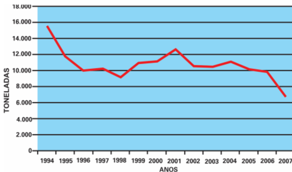
Figura 4 - Produção anual do caranguejo Ucides cordatus no Brasil, nos período de 1994 a 2007.
